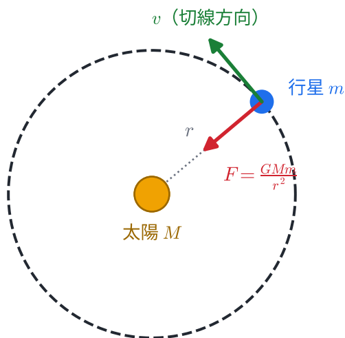
圖 2-5：圓軌道上，萬有引力 F = GMm/r^2 （指向太陽）正好扮演向心力的角色，使行星持續轉向；速度 v 永遠沿軌道切線方向。
